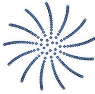
Golden Angle + 1° 138.508...°
