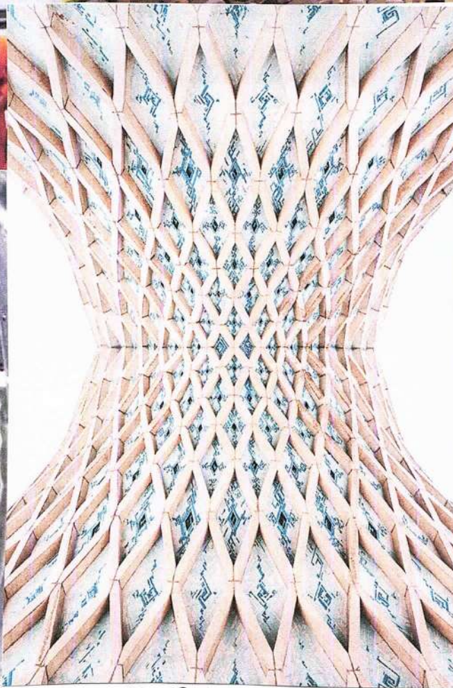
HYPERBOLA
