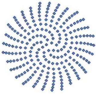
Golden Angle - 1° 136.508...°
