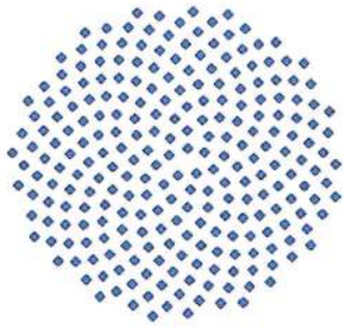
Golden Angle 137.508...°
