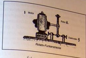
Éclateur d'étincelles rotatif
