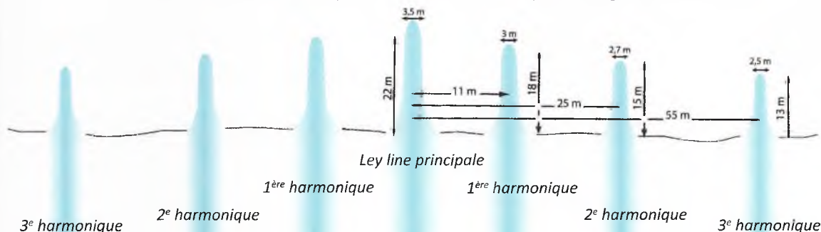
Dessin en coupe d'une Ley line Marie de niveau 1
